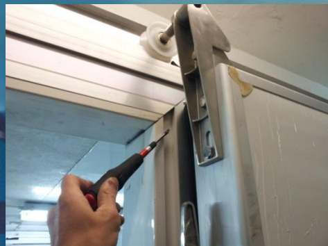
趟門路軌 Door Rail
